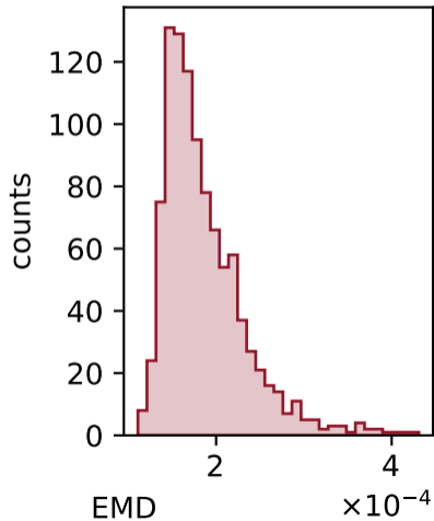
FFT
