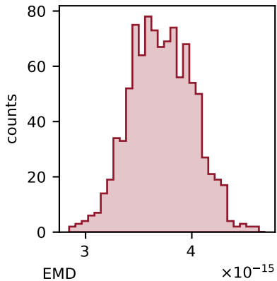
FFT
